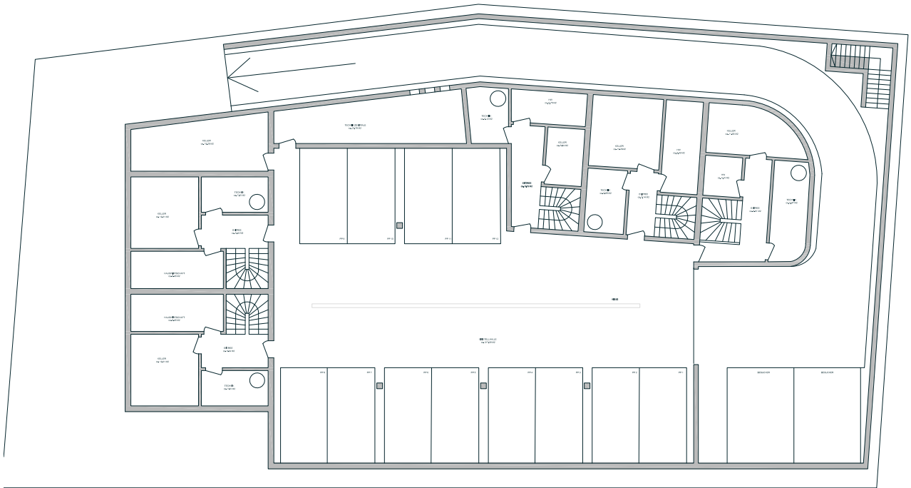
UNTERGESCHOSS
