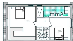
DACHGESCHOSS
